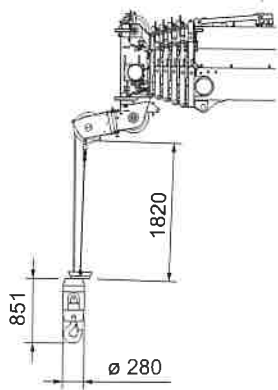
5.6ton フック
